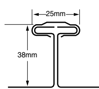
38mm Batten Cap T Seam S-5-T, S-5-T Mini
