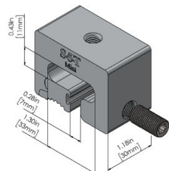
S-5-T™ Mini
