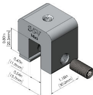
S-5-V™ Mini
