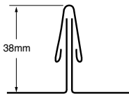
38mm Batten Cap S-5-N, S-5-N Mini
