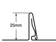
25mm Snap Seam S-5-S, S-5-S Mini
