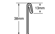
38mm Double Fold S-5-E, S-5-E Mini
