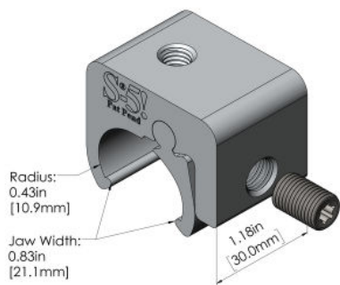
S-5-ZH™ Mini
