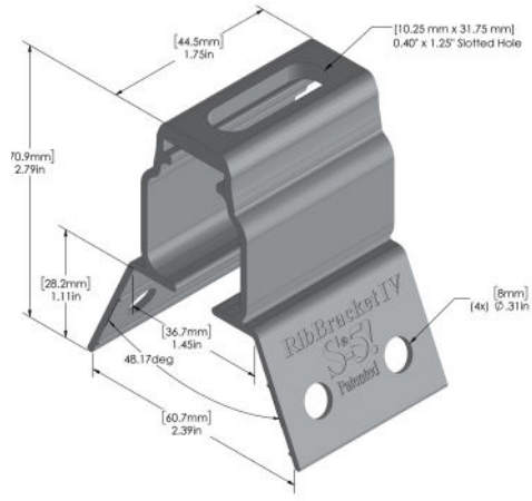
RibBracket™ IV
