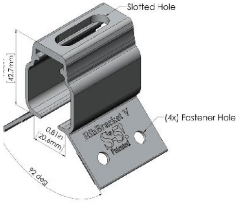
RibBracket™ V
