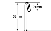
38mm Double Fold S-5-V, S-5-V Mini S-5-U, S-5-U Mini
