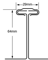
64mm Batten Cap T Seam S-5-T, S-5-T Mini
