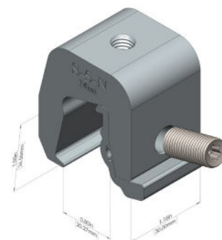
S-5-N™ Mini
