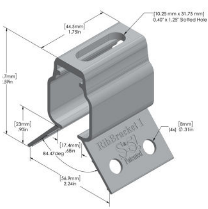
RibBracket™ I
