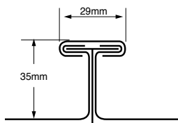
35mm T Seam S-5-T, S-5-T Mini
