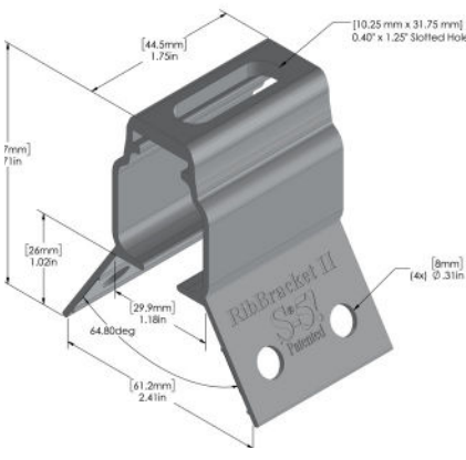
RibBracket™ II
