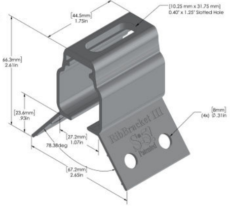
RibBracket™ III
