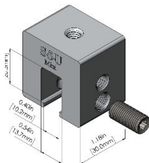
S-5-U™ Mini
