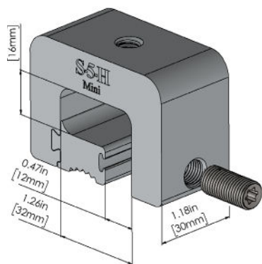
S-5-H™ Mini
