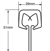
51mm Bulb Seam Cap S-5-Q, S-5-Q Mini
