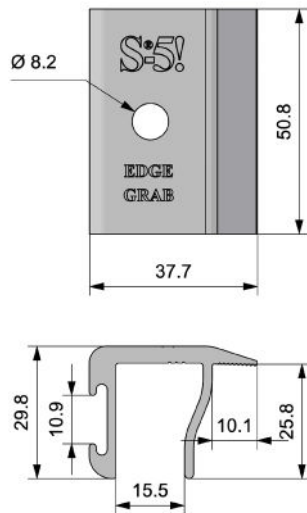
PV 2.0 EdgeGrab
