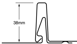
38mm Nail Strip S-5-N 1.5, S-5-N 1.5 Mini
