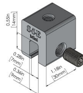
S-5-E™ Mini
