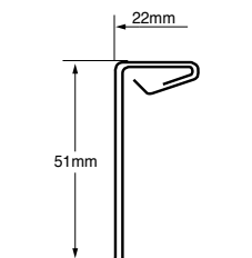
51mm Single Fold S-5-H90, S-5-H90 Mini S-5-U, S-5-U Mini S-5-H, S-5-H Mini
