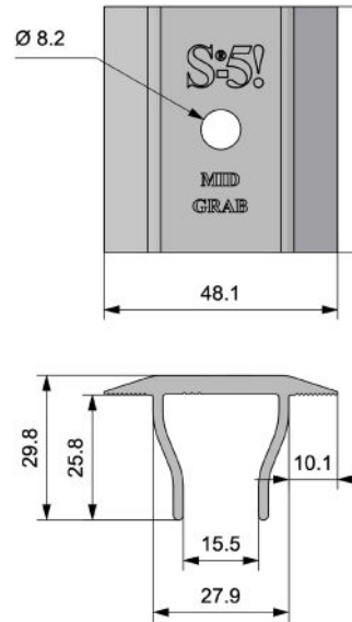
PV 2.0 MidGrab
