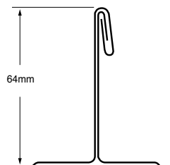
64mm Double Fold S-5-V, S-5-V Mini S-5-U, S-5-U Mini
