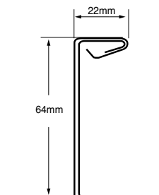
64mm Single Fold S-5-H90, S-5-H90 Mini S-5-U, S-5-U Mini S-5-H, S-5-H Mini
